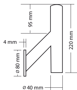
Wandausführung » gerade «
