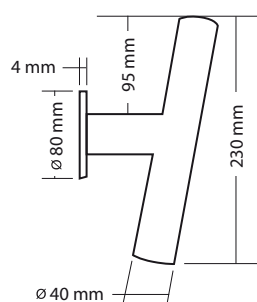
Wandausführung » Fackel «
