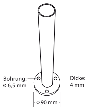
Montageplatte
