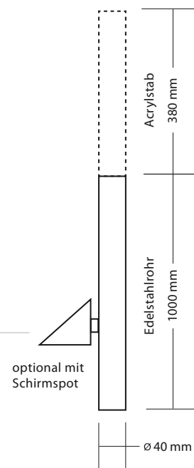
Standardausführung
